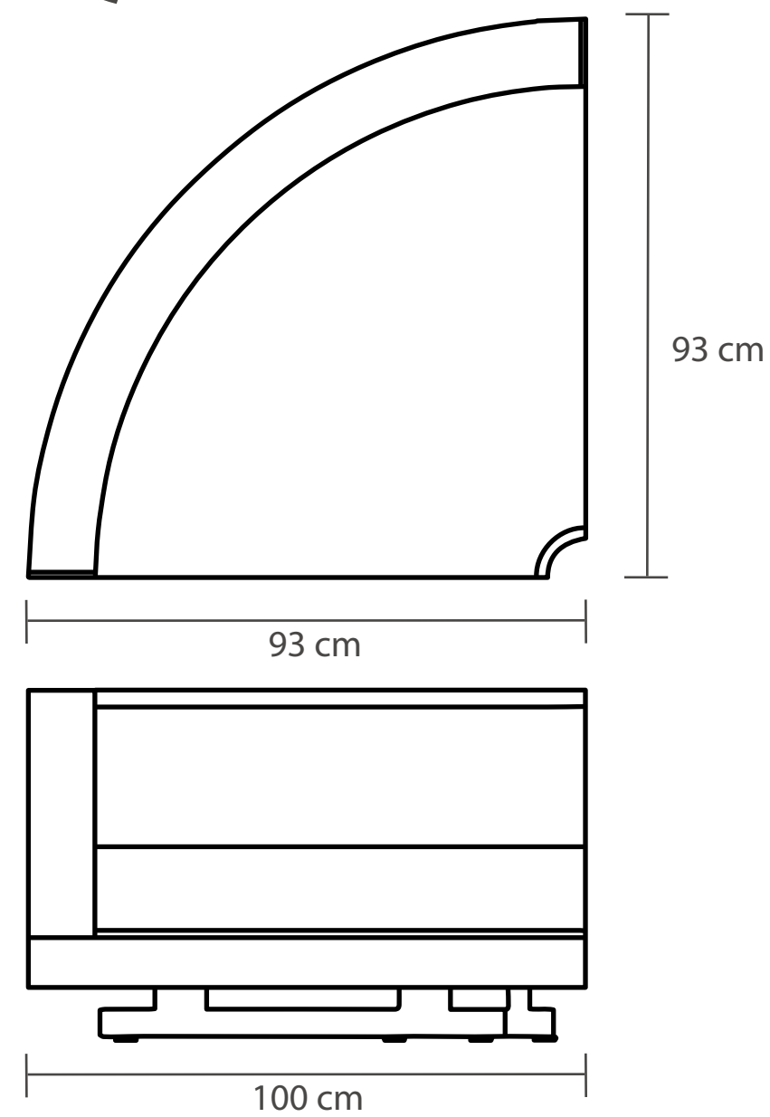
ESQUINERO CURVO
